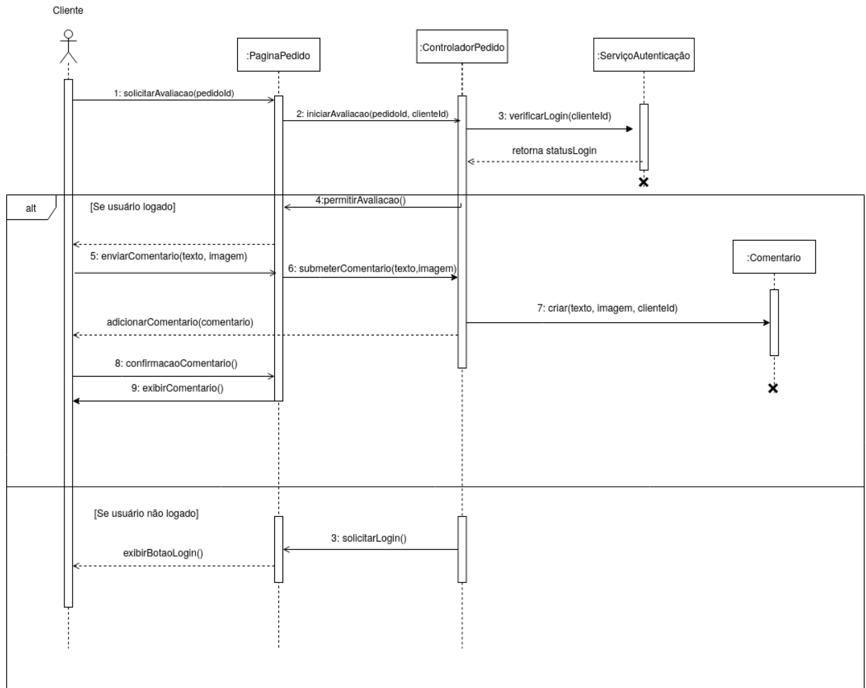
Imagem 6 - Diagrama de Sequência: UC-3 - Avaliar produto e gerir feedback
