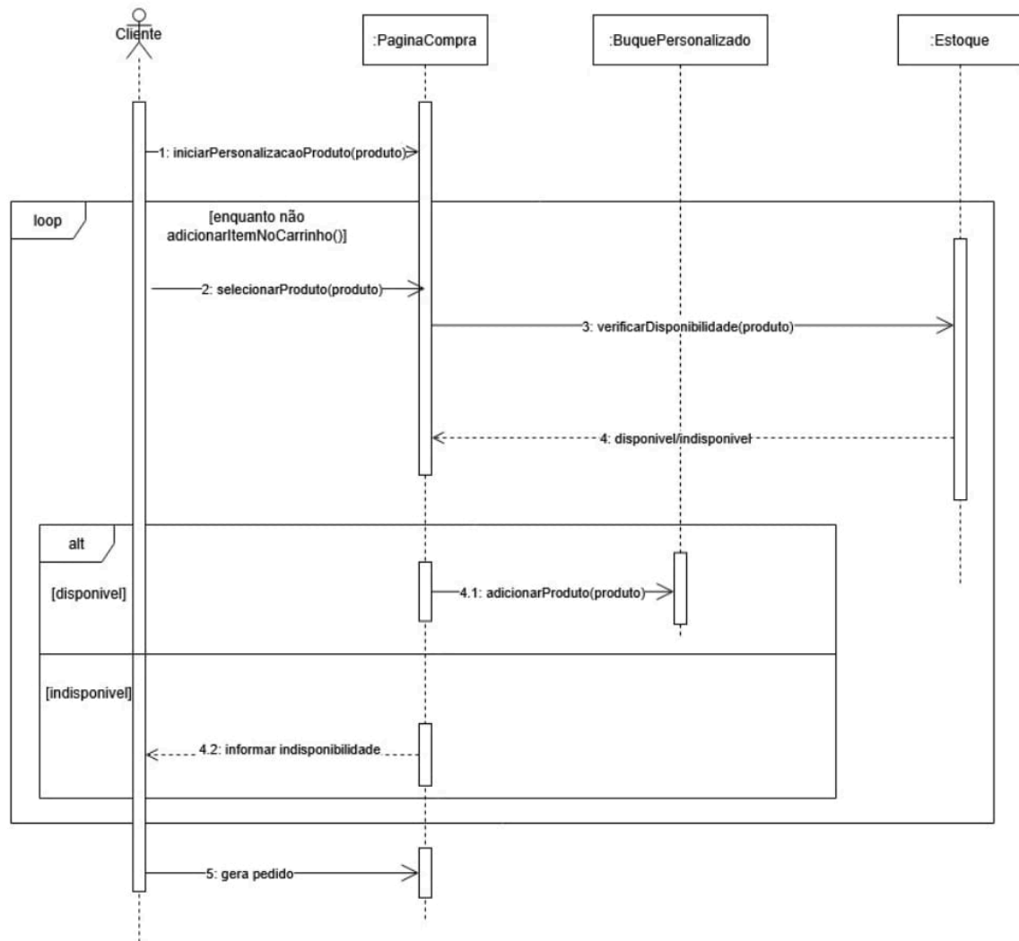
Imagem 9 - Diagrama de Sequência: UC-6 - Montar Buquê Personalizado
