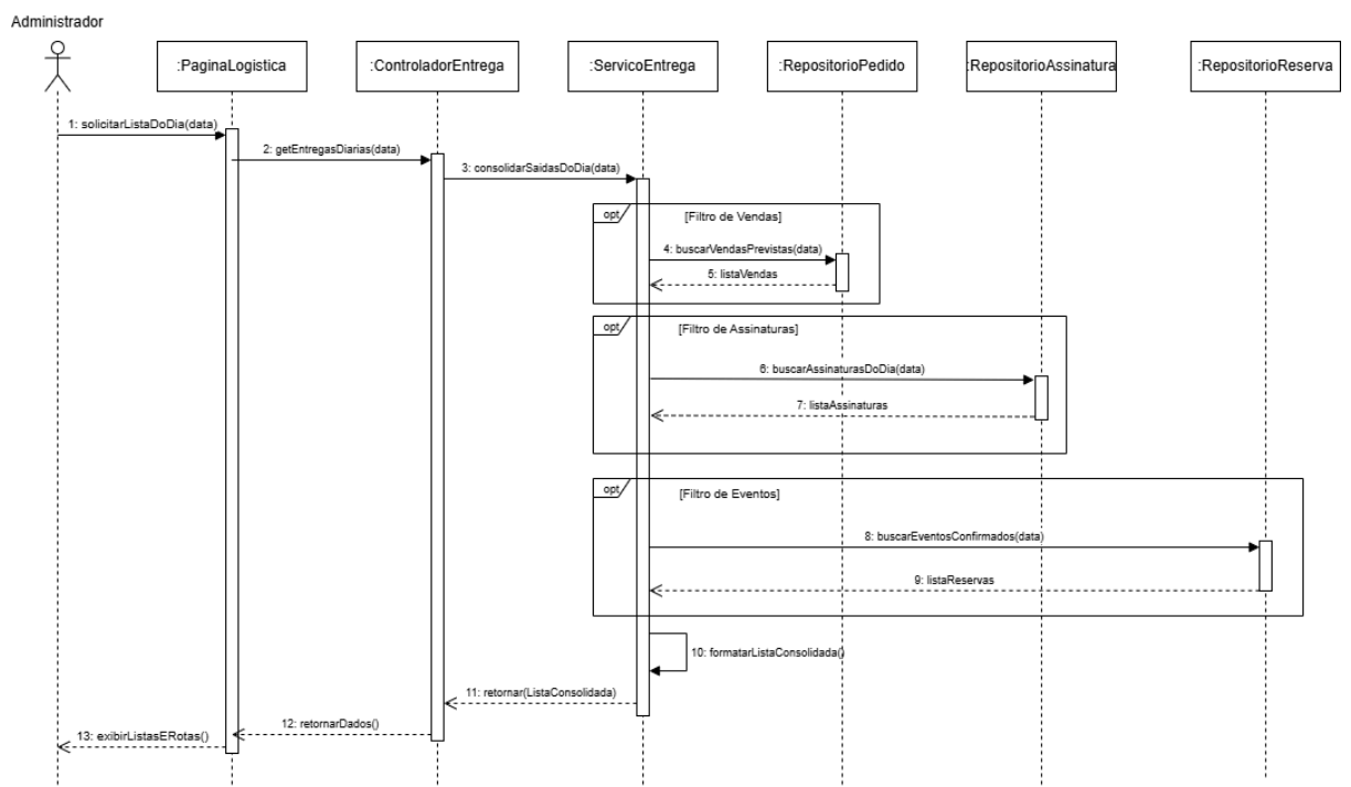
Imagem 8 - Diagrama de Sequência: UC 05 - Controle de entregas diárias
