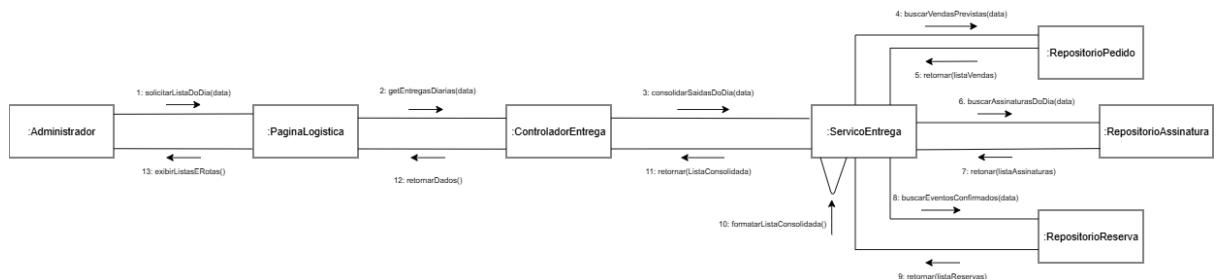
Imagem 14- Diagrama de Interação (Comunicação) da operação solicitar Lista do dia do Caso de Uso 5 – Controle de entregas diárias
