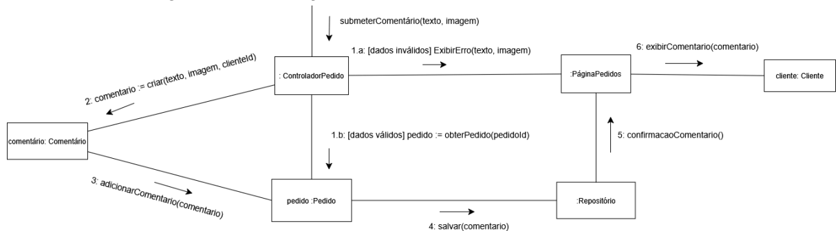
Imagem 12 - Diagrama de Interação (Comunicação) da operação submeter comentário do Caso de uso 3 – Avaliar produto e gerir feedback.
