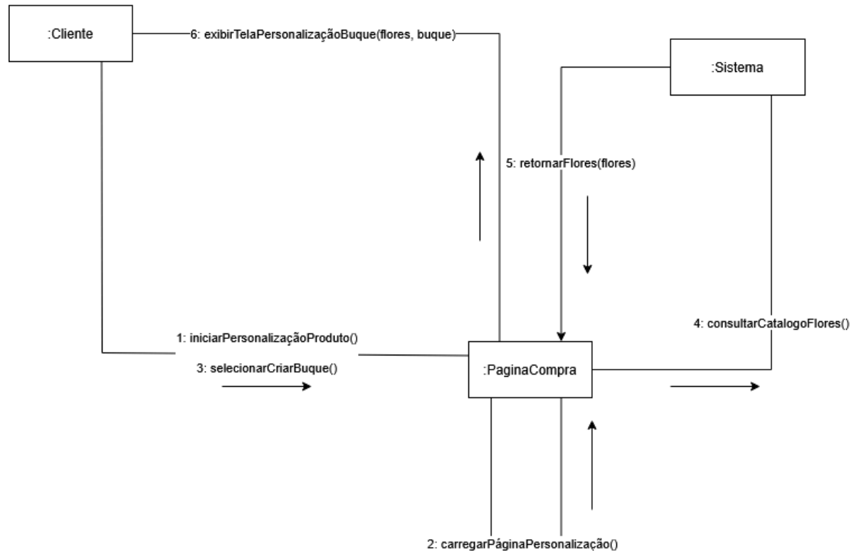
Imagem 16- Diagrama de Interação (Comunicação) da operação iniciar personalização do produto do Caso de Uso 6 – Montar buquê personalizado
