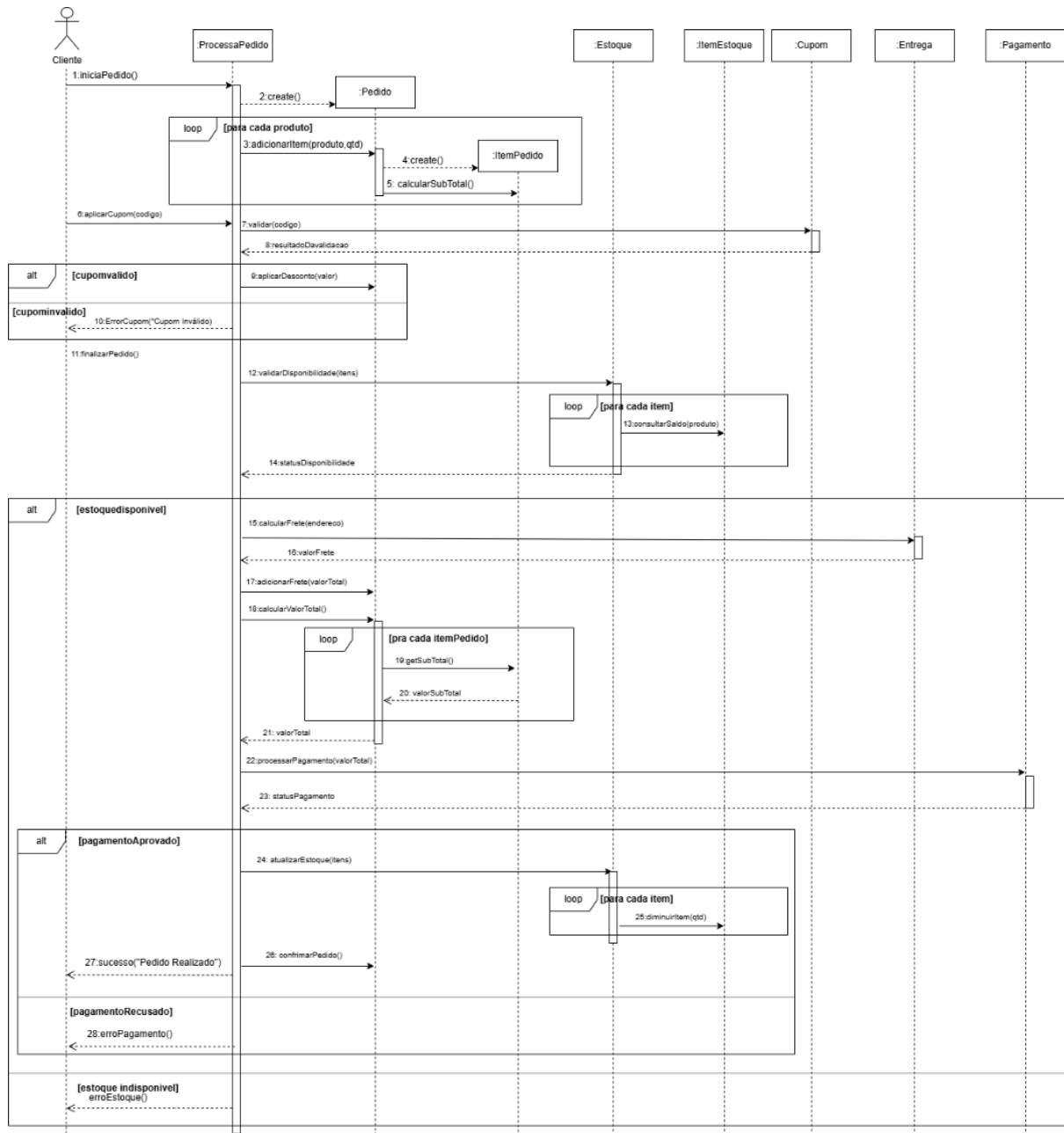
Imagem 4 - Diagrama de Sequência: UC-1 - Realizar Pedido
