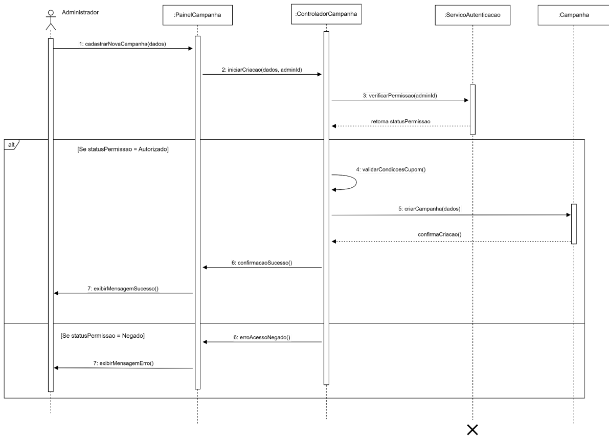
Imagem 7 - Diagrama de Sequência: UC-4 - Criar Campanha Promocional
