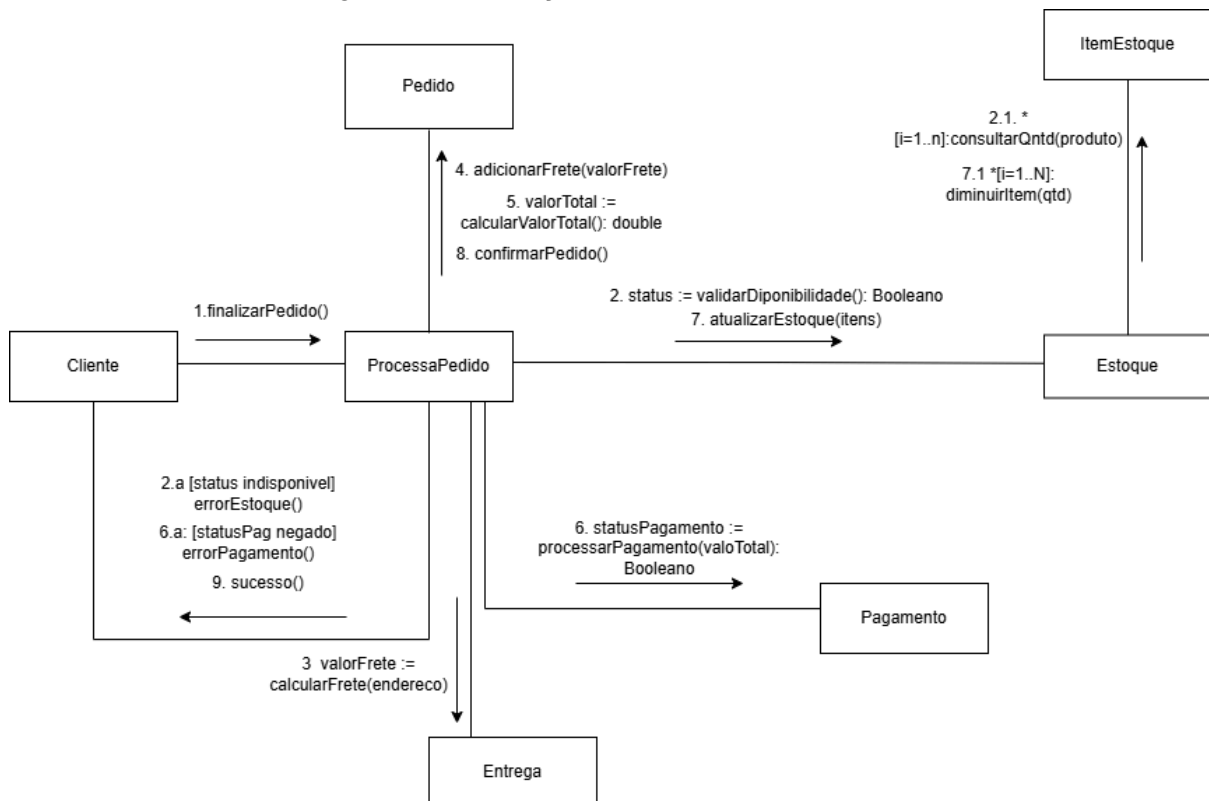
Imagem 10 – Diagrama de Interação (Comunicação) da operação finalizar pedido do caso de Uso 1 – Realizar vendas.
