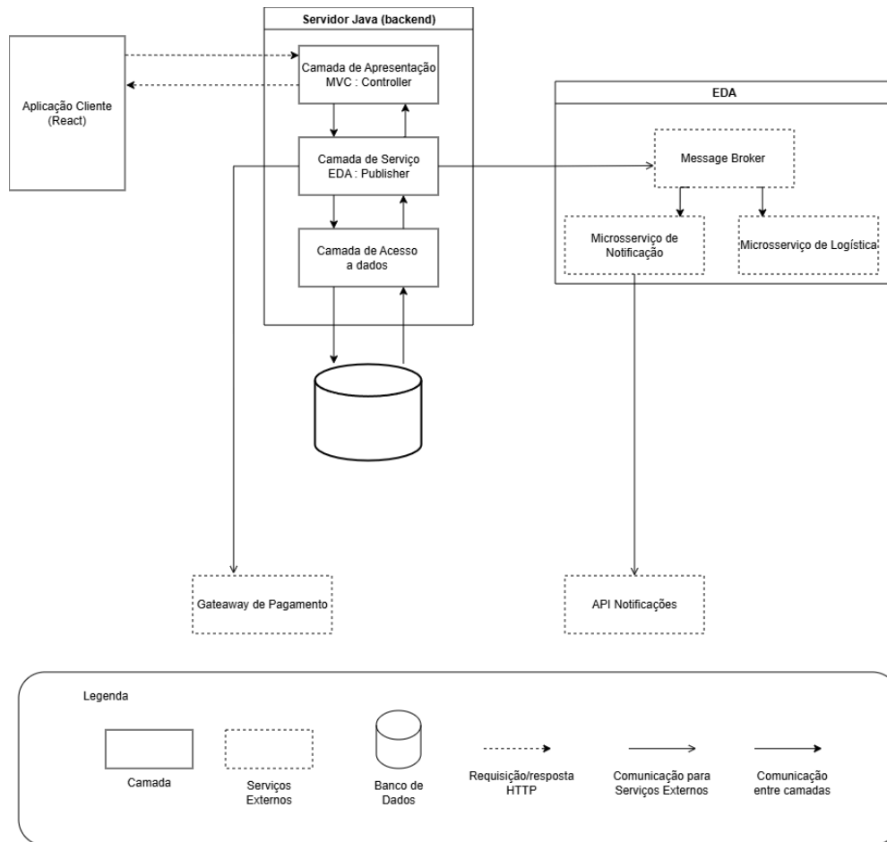
Imagem 1 - Diagrama de Visão Arquitetural.
